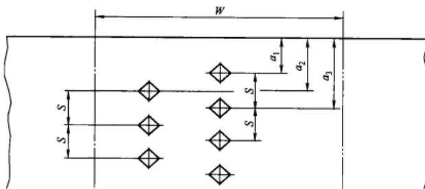
图 1 硬度压痕的位置
