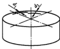
图2 硬度测量点的位置
